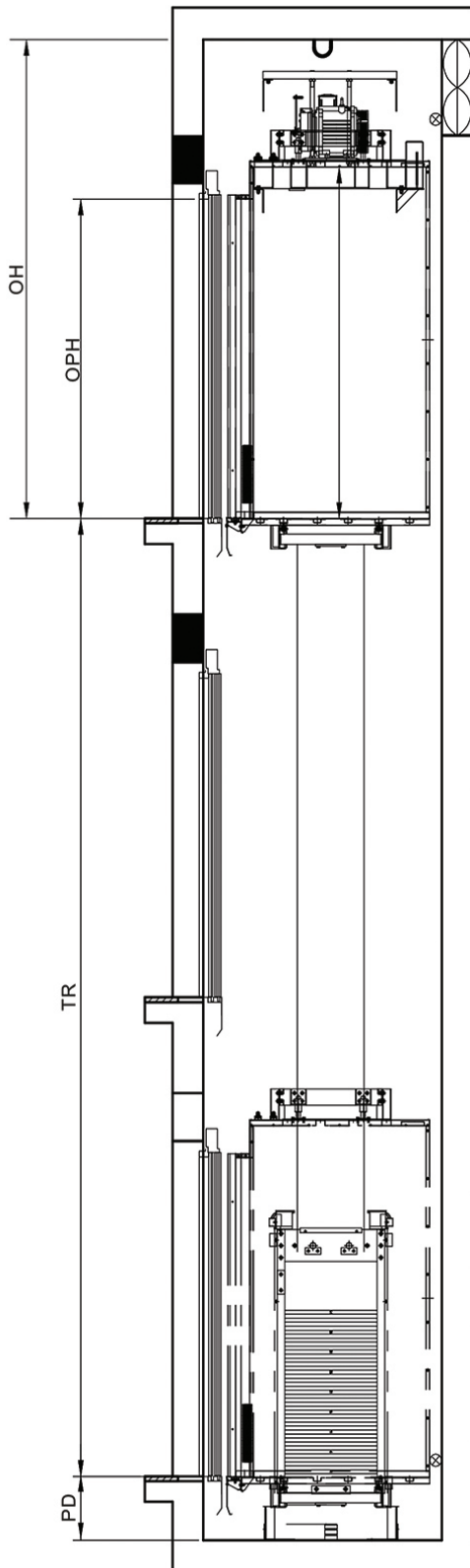
Hoistway Elevation
